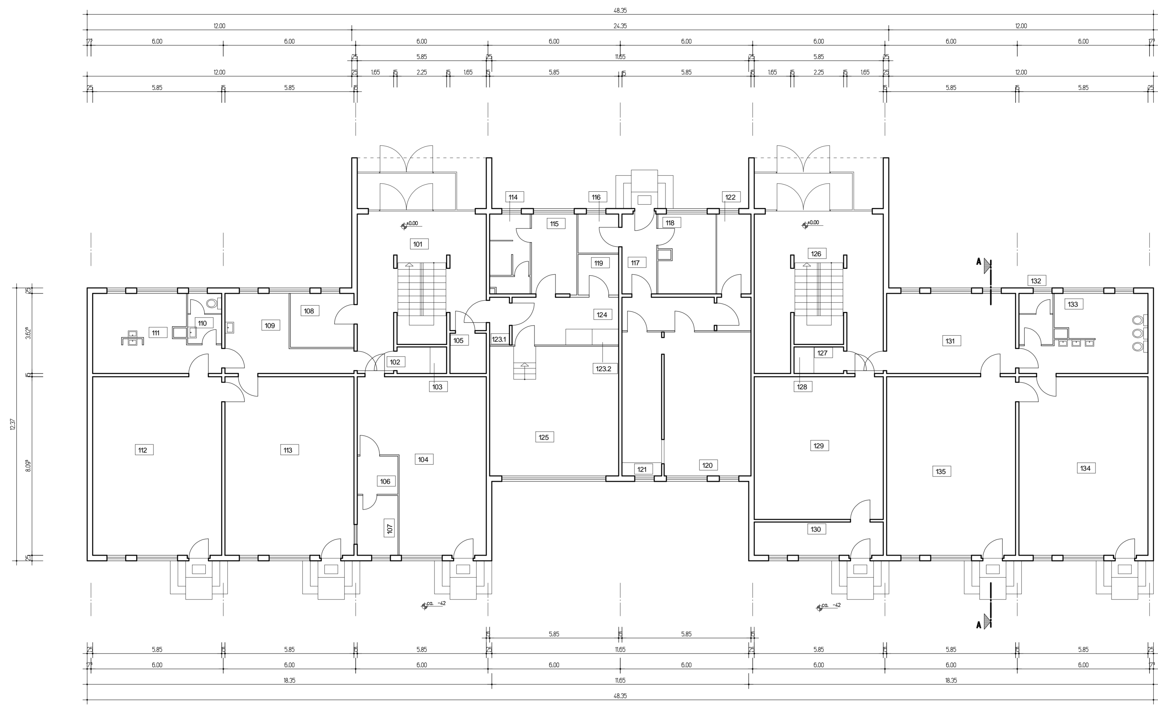
GRUNDRISS ERDGESCHOSS (BESTAND) M 1:100
