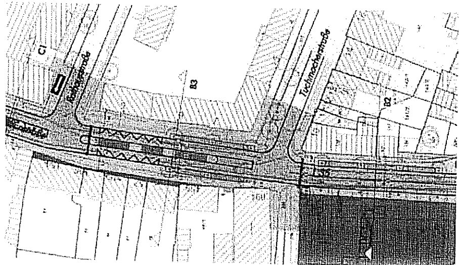
Abbildung 89 Lageplan Abschnitt B3 Var. A „Bushaltestellen“
