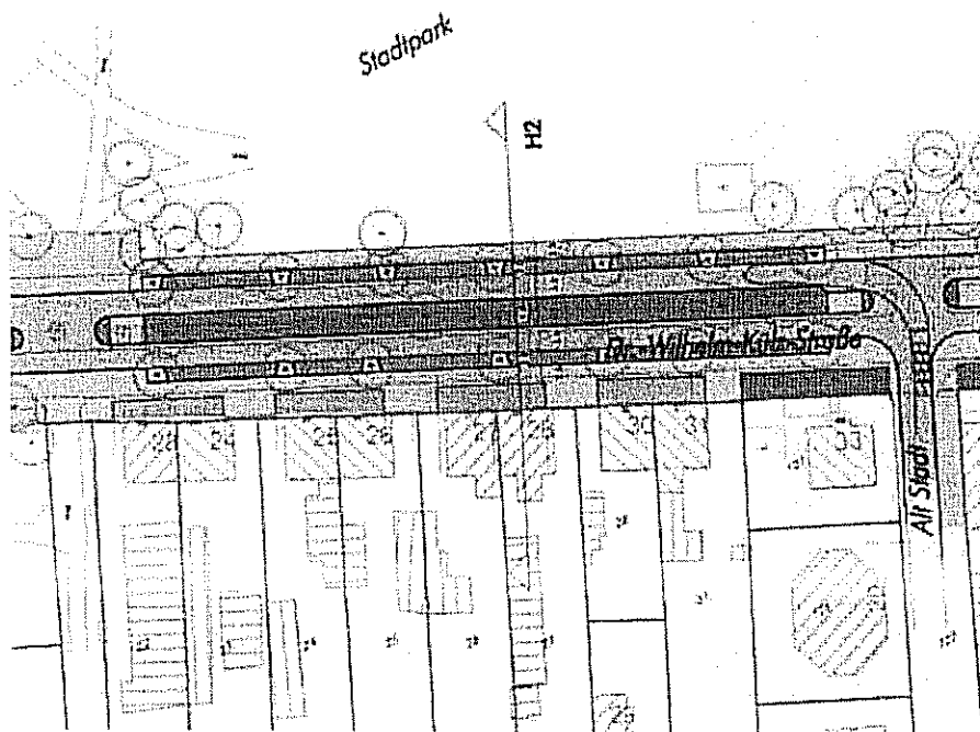
Abbildung 115 Lageplan Abschnitt H2
