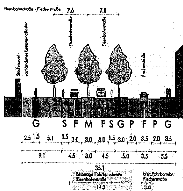
Abbildung 83 Querschnitt B1.1 Var A
