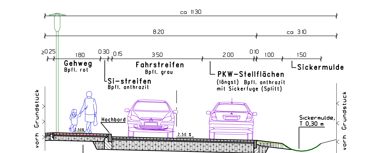
Straßenquerschnitt -Variante 2B-
